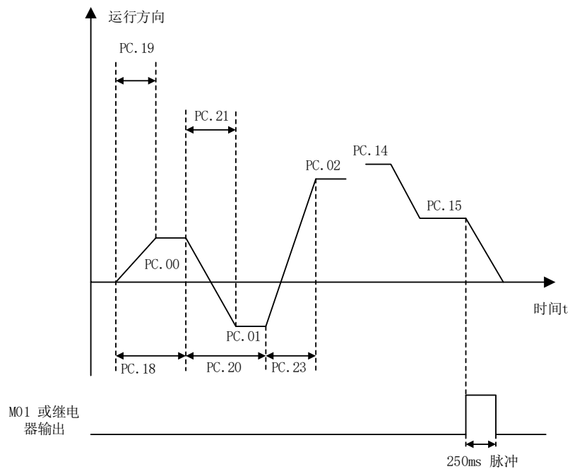
图 4-29 简易 PLC 示意图
