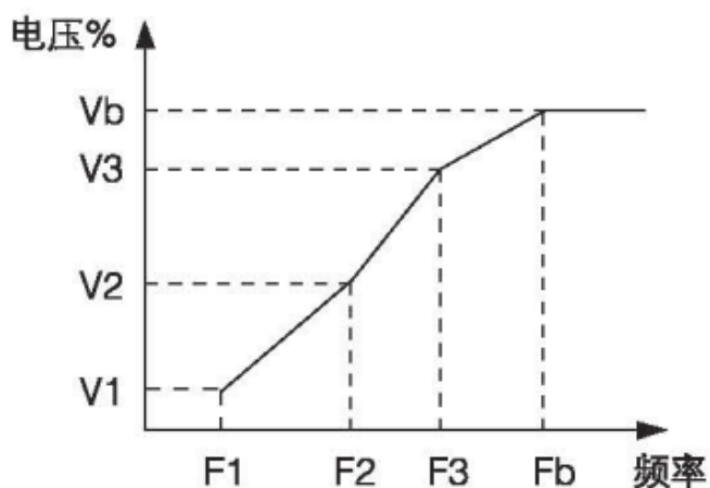
图 4-3 多点 V/F 曲线设定示意图
