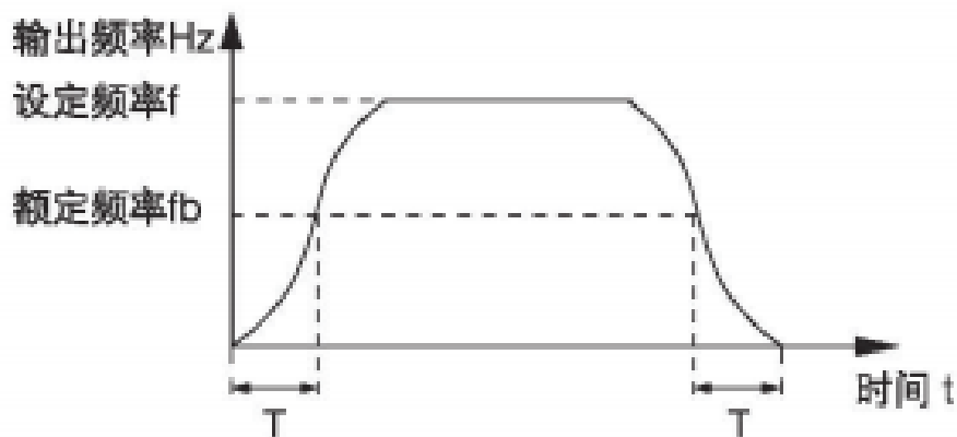
图 4-10 S 曲线加减速 B 示意图
