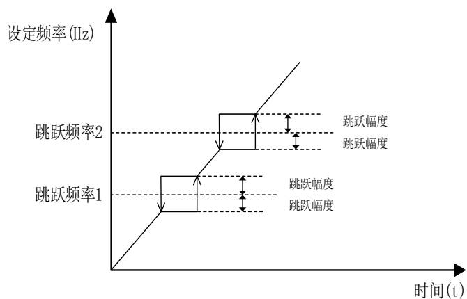
图 4-17 加减速过程中跳跃频率有效示意图
