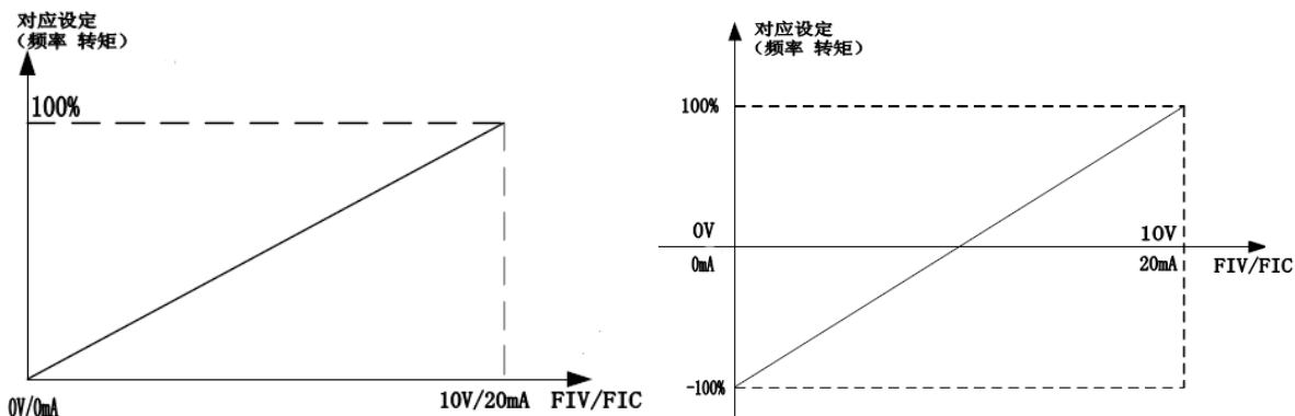
图 4-9 模拟给定与设定量的对应关系
