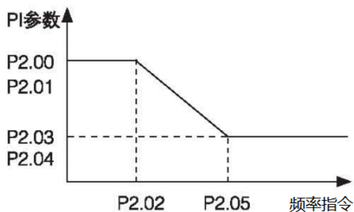
图 4-1 PI 参数示意图
