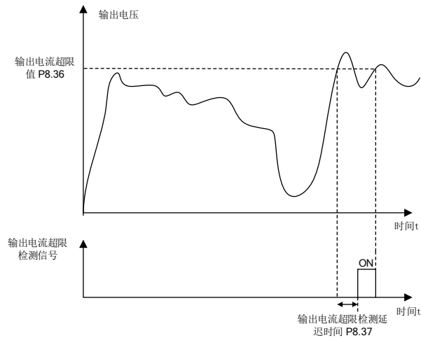
图 4-21 输出电流超限检测示意图
