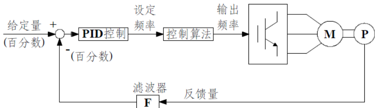
图 4-23 过程 PID 原理框图
