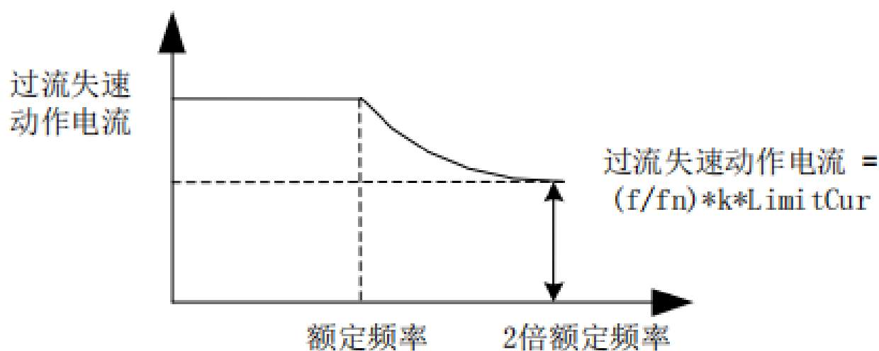
图 4-5 倍速过流失速动作示意图
