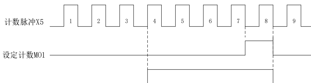
图 4-28 设定计数值给定和指定计数值给定示意图
