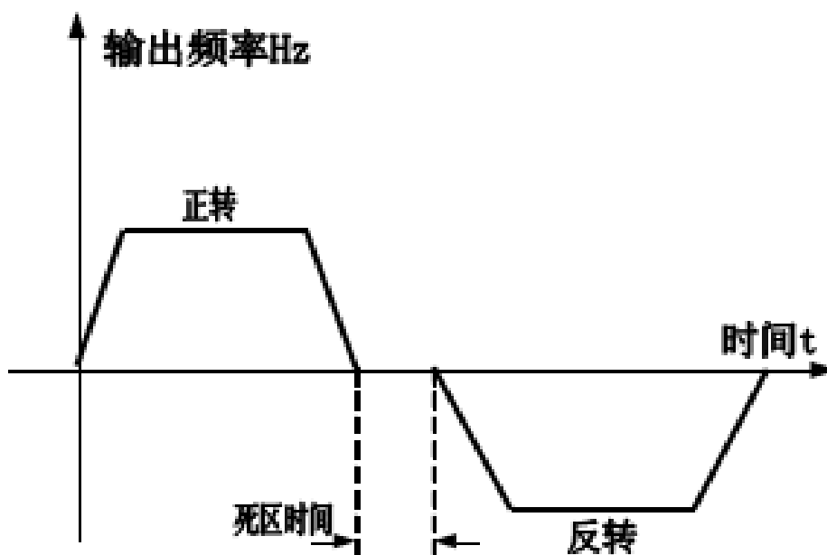
图 4-14 正反转死区时间示意图
