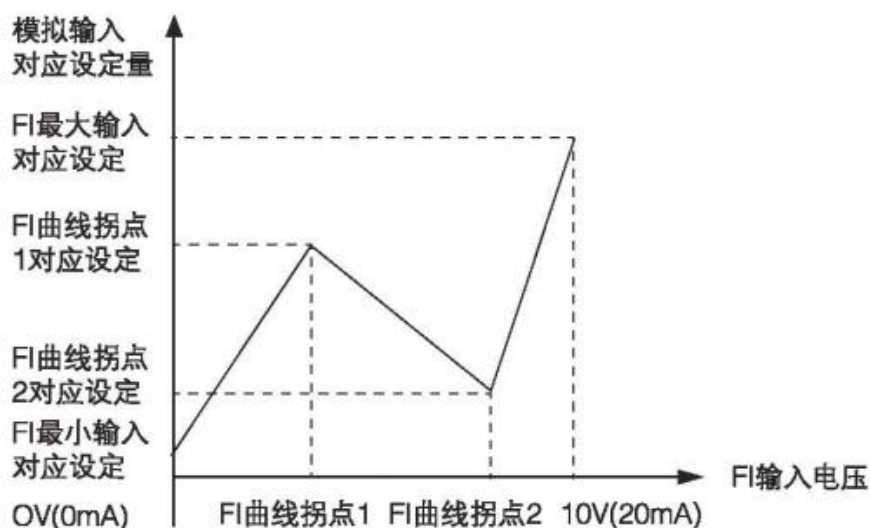
图 4-30 曲线 4 和曲线 5 示意图
