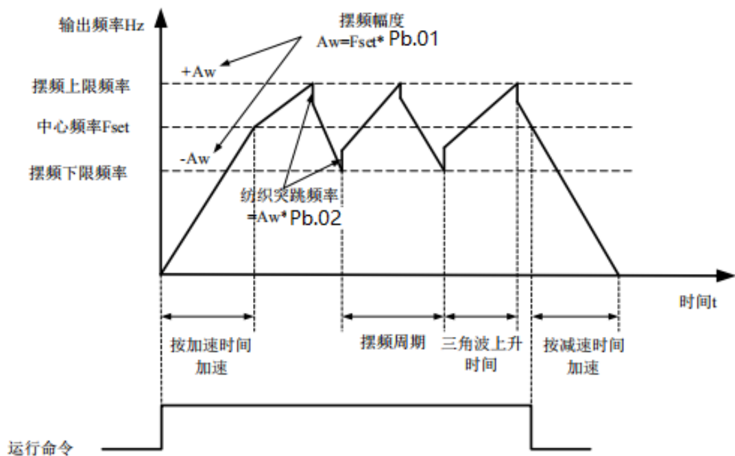
图 4-27 摆频工作示意图
