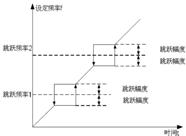
图 4-13 跳跃频率示意图
