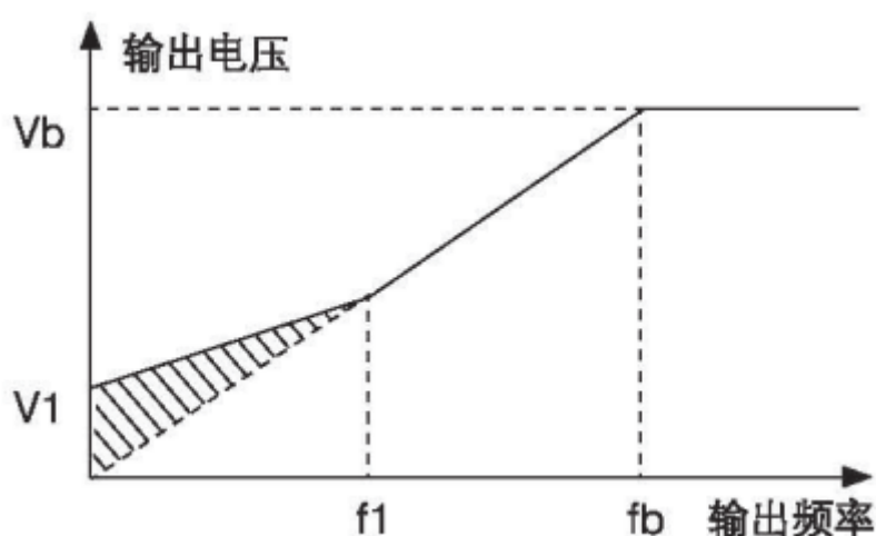
图 4-2 手动转矩提升示意图
