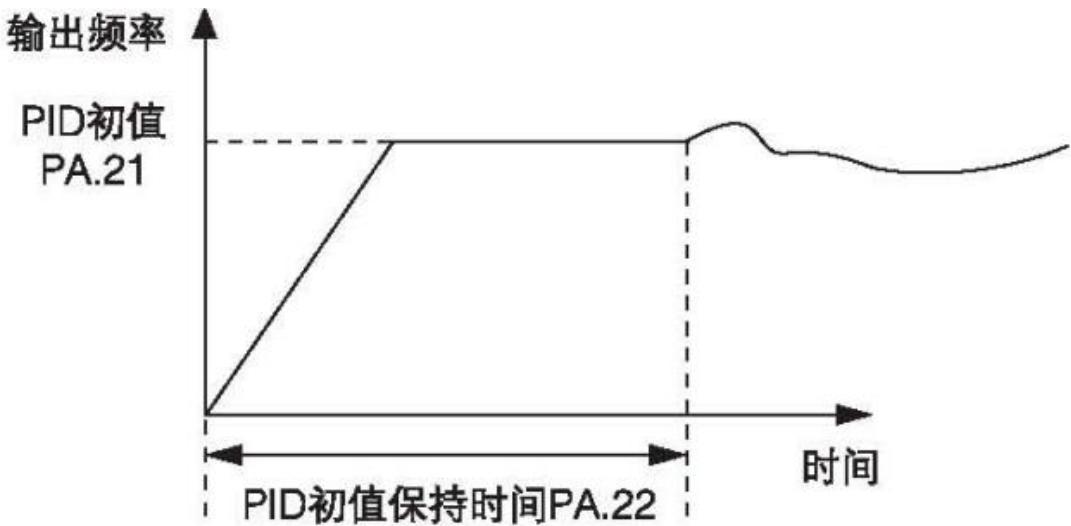
图 4-26 为 PID 初值的功能示意图。
