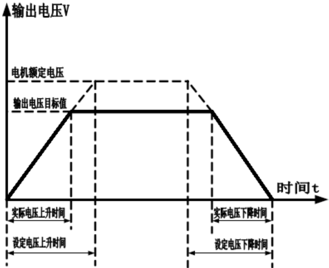
图 4-4 V/F 分离示意图
