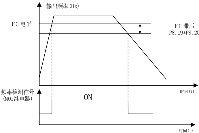
图 4-15 FDT 电平示意图
