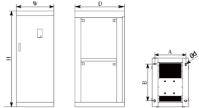
壁挂机安装示意图
