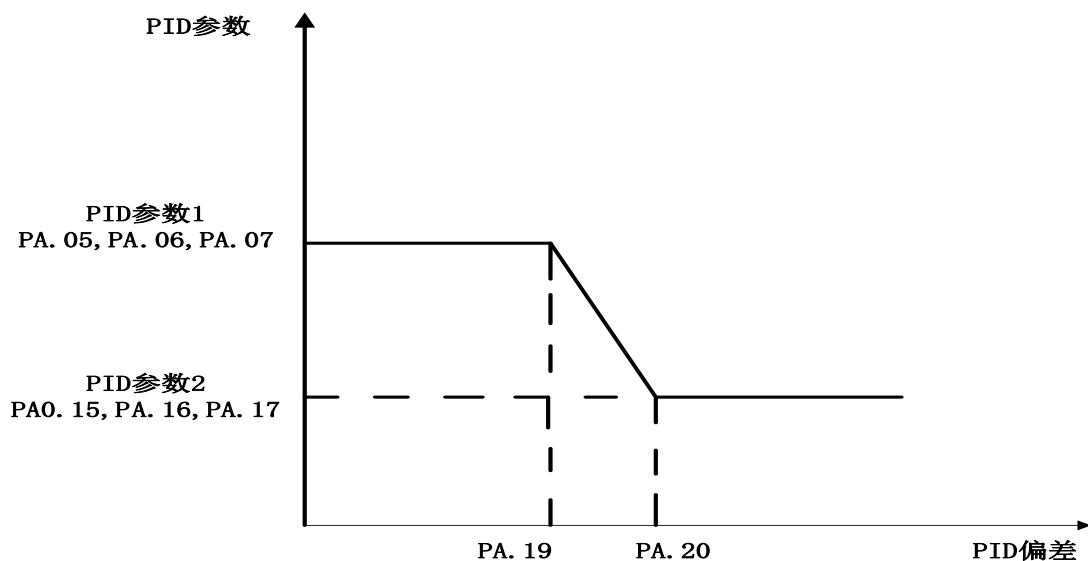
图 4-25 PID 参数切换
