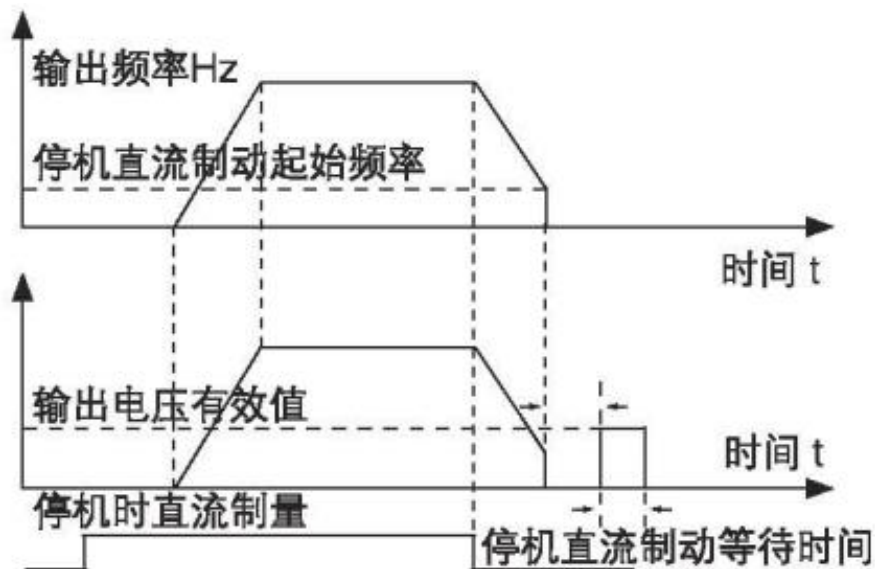
图 4-12 停机直流制动示意图
