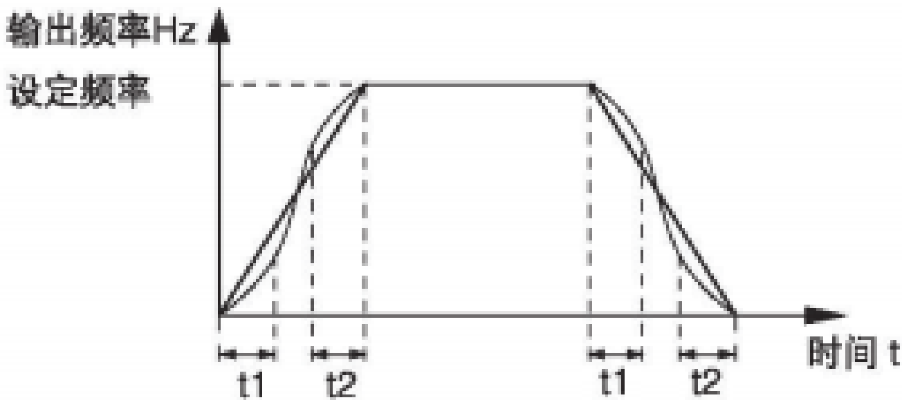
图 4-11 S 曲线加减速 A 示意图
