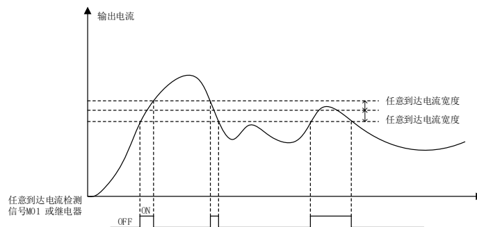
图 4-22 任意到达电流检测示意图
