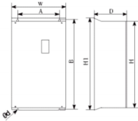
柜式机安装示意图
